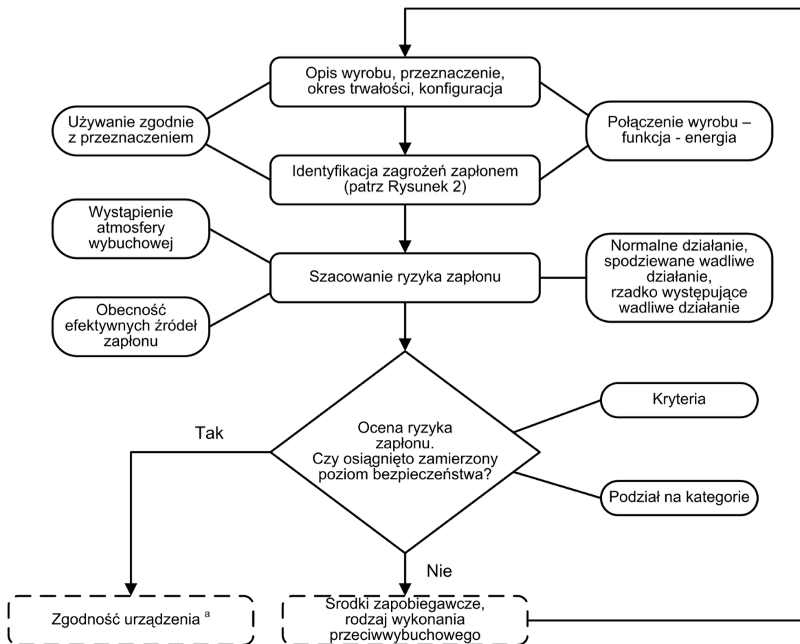
Rysunek 4: Schemat procedury oceny ryzyka zapłonu.
