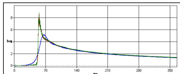
Rys. 5. Przebieg ciśnień wybuchu we wnętrzu silnika w ruchu
